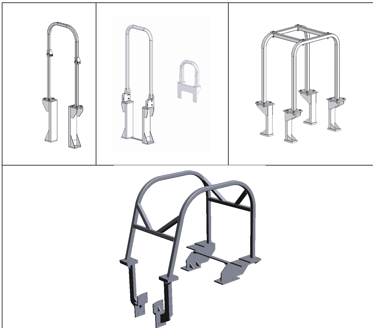
Figura 10. Veduta d'insieme delle strutture di protezione a due montanti posteriori, a due montanti anteriori, a quattro montanti ► R2 ed a quattro montanti a profilo compatto (CROPS) ◀
