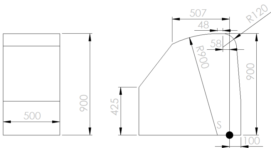
►R2 Figura 3. Volume di sicurezza per struttura di protezione a quattro montanti a profilo compatto. Dimensioni in mm ◀
