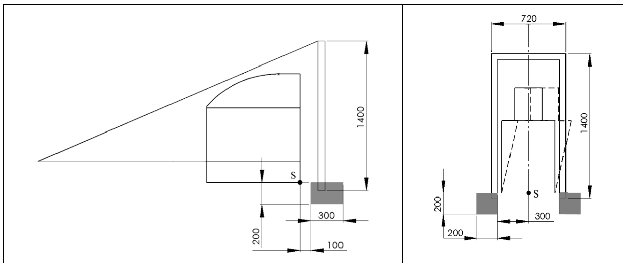
Figura 8. VUC (area ombreggiata) per telai di protezione a due montanti posteriori, vista laterale e posteriore (dimensioni in mm)*.
