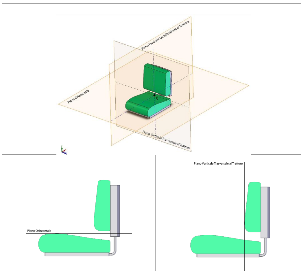
Figura 4. Individuazione del punto S del sedile
