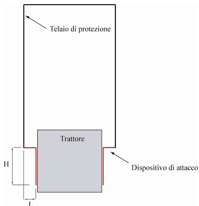
Figura 5. Conformazione e principali dimensioni del dispositivo di attacco
