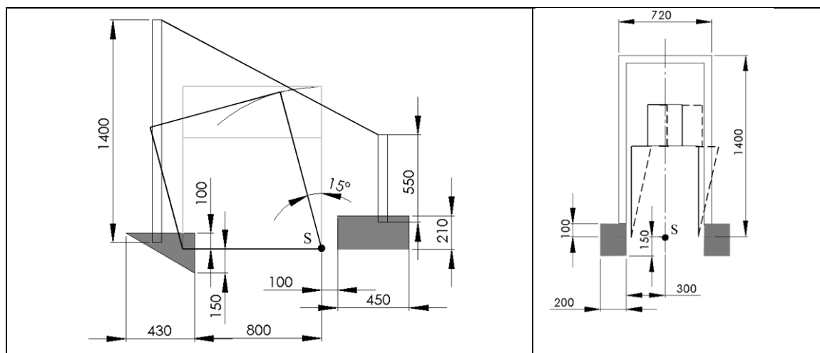
Figura 7. VUC (area ombreggiata) per telai di protezione a due montanti anteriori, vista laterale e posteriore (dimensioni in mm)*.
