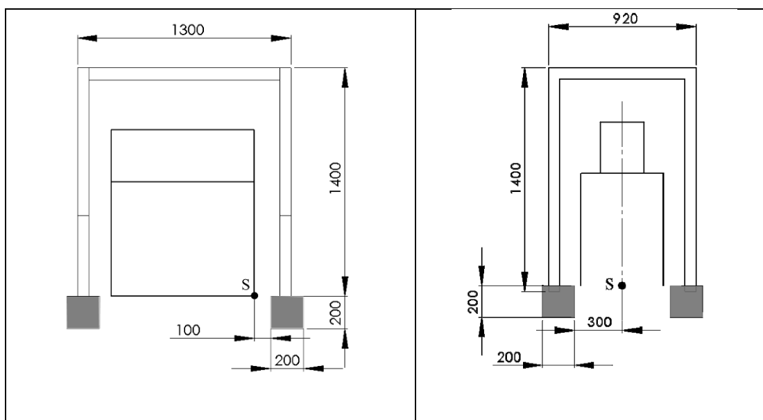
Figura 6. VUC (area ombreggiata) per telai di protezione a quattro montanti, vista laterale e posteriore (dimensioni in mm)*.
