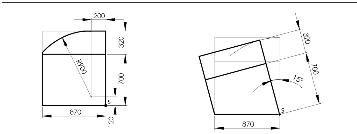
Figura 2. Volume di sicurezza per struttura di protezione a due montanti posteriore (a sinistra) ed anteriore (a destra). Dimensioni in mm
