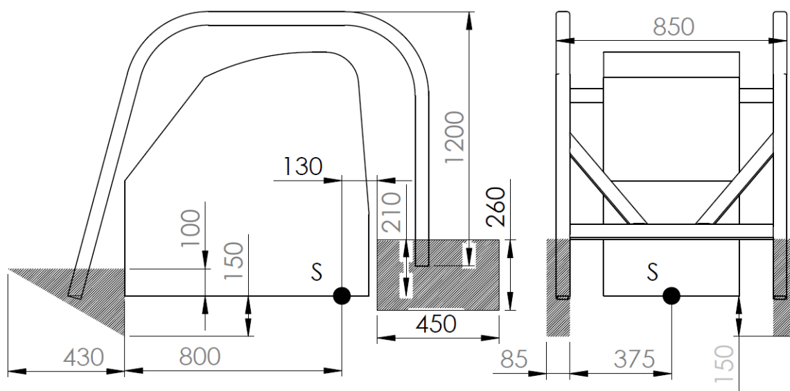
► R2 Figura 9. VUC (area ombreggiata) per telai di protezione a quattro montanti a profilo compatto (CROPS), vista laterale e posteriore (dimensioni in mm) ◀
