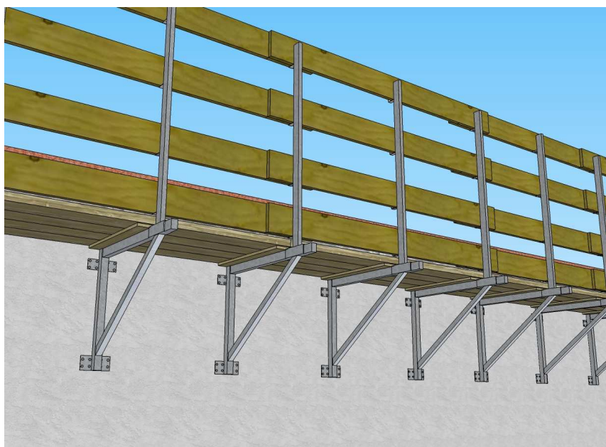
Fig. 5 – Parapetto a mensola
